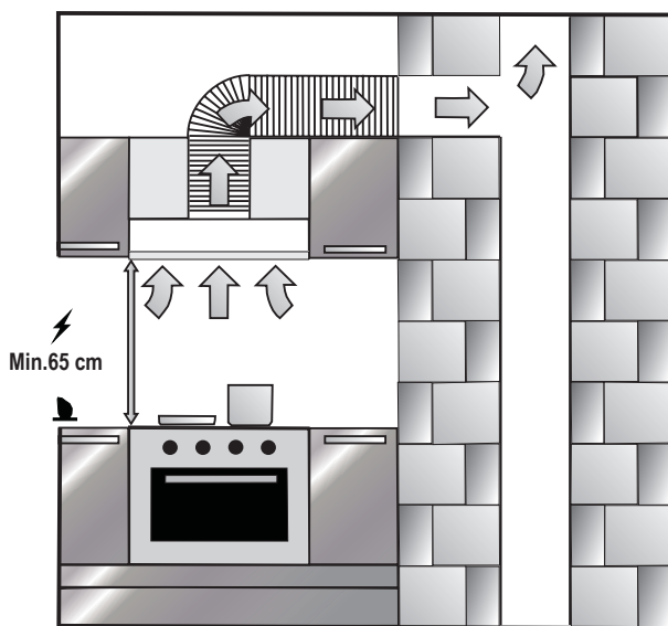
Rys. 7: Instalacja urządzenia
